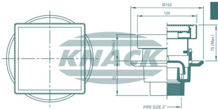
FLOOR DRAIN (หน้าสแตนเลสสตีล) แบบดักสับ MODEL : 227 B (ขนาด 2")
