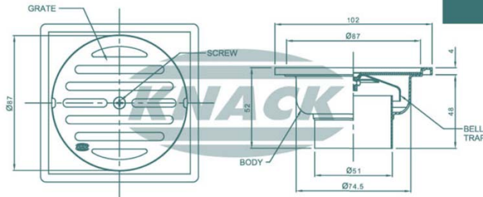
FLOOR DRAIN MODEL : 312 S (สำหรับ PVC ยูน 2"-3")
