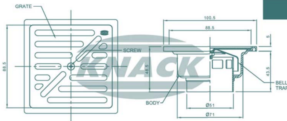
FLOOR DRAIN MODEL : 300 Z (สำหรับ PVC ยูน 2"-3")
