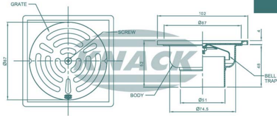
FLOOR DRAIN MODEL : 303 S (สำหรับ PVC ยูน 2"-3")
