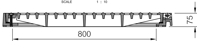
SECTION B-B SCALE 1 : 10
